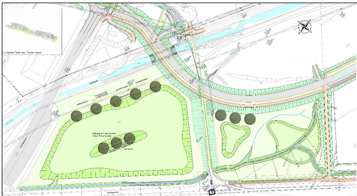
Abbildung 20: Gestaltungsplan Retentionsfläche; Zink Ingenieure, 29.03.2019
