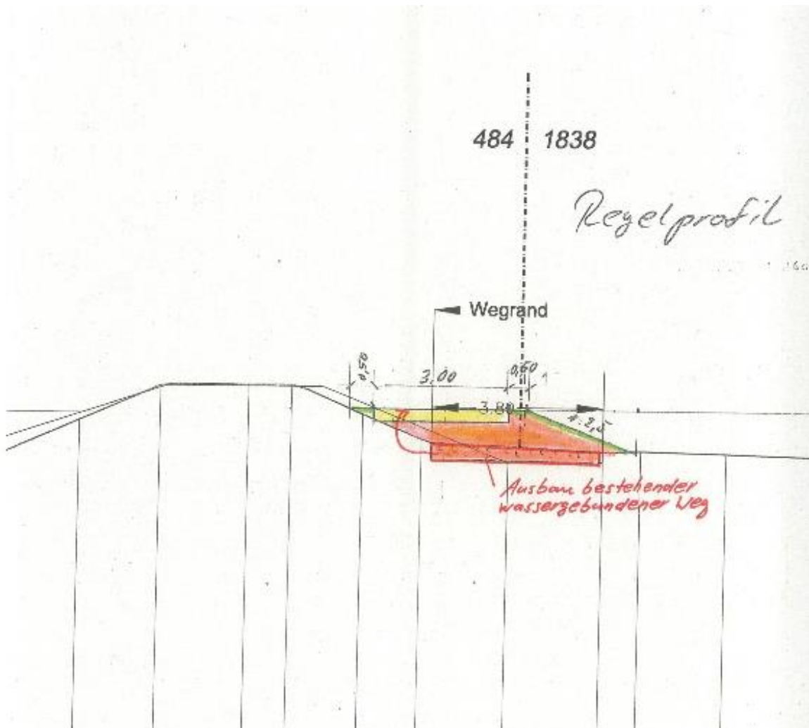
Abbildung 7: Regelquerschnitt mit bestehender und geplanter Lage des Wirtschaftsweges
